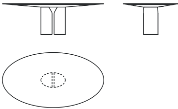
oval table L250 D130 H74 cm base L60 D36
